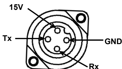
Rysunek 1 Rozmieszczenie zacisków w gnieździe przyłączeniowym RS-232 i ładowania akumulatora (widok od frontu)
